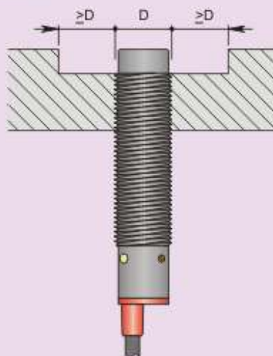
Montaggio sporgente
